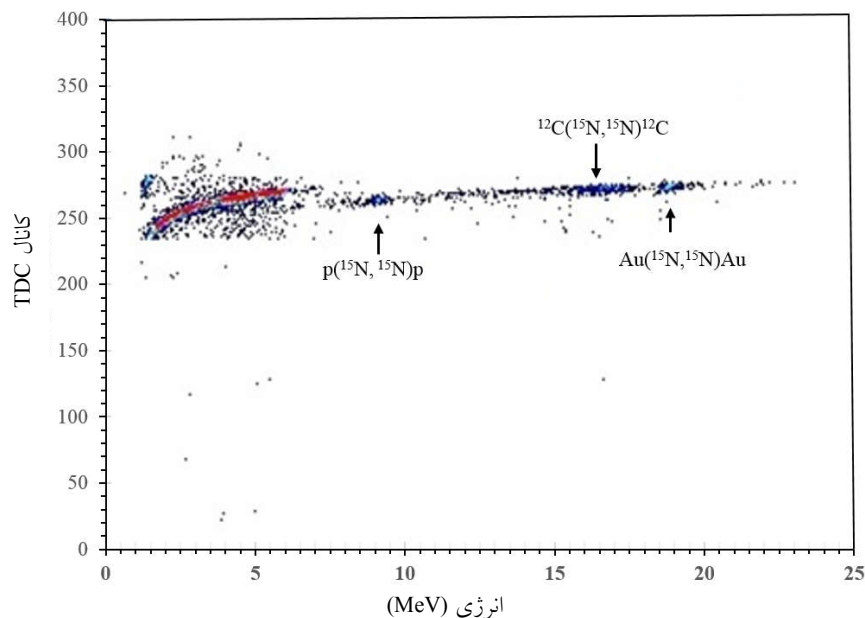
شکل ۲. (رنگی در نسخه الکترونیک) طیف انرژی حاصل از برهم‌کنش بین هسته ^{15}\text{N} و هدف \text{CH}_7 (Au) در زاویه 17^\circ ، محور افقی انرژی و محور عمودی زمان پرواز بر حسب نانوثانیه.
