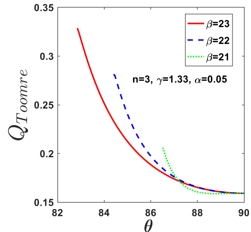
شکل ۵. (رنگی در نساخه الکترونیکی) رفتار زاویه‌ای پارامتر تومره برای مقادیر مختلف آهنگ سرمایش.
