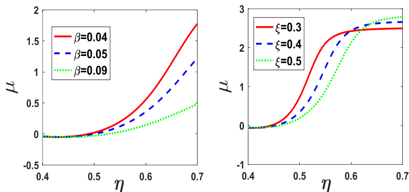
شکل ۵. (رنگی در نسخه الکترونیکی) راه حل‌های خودمشابهی وابسته به زمان برای عدد ماخ. پارامترهای ورودی برای هر دو نمودار به صورت \alpha = 0.06 ، \gamma = 1/33 و f = 0.07 ، \dot{m} = 0.01 است. نمودار سمت راست: خط پر رنگ ( \xi = 0.3 )، خط چین ( \xi = 0.4 ) و خط نقطه چین ( \xi = 0.5 ) اثرات وشکسانی شعاعی را روی عدد ماخ را نشان می‌دهد. نمودار سمت چپ: خط پر رنگ ( b = 0.04 )، خط چین ( b = 0.05 ) و خط نقطه چین ( b = 0.09 ) اثرات پارامتر مغناطیسی را روی عدد ماخ نشان می‌دهد.
