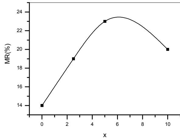
شکل ۱۰. نمودار MR برای نمونه‌های \text{LSMO}/x\text{ppy} در میدان 8000 اورستد و در دمای 77 کلوین.
