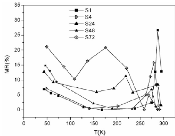
شکل ۳۳. تغییرات مغناطومقاومت نمونه‌های \text{La}_{x/8}\text{Sr}_{7/8}\text{MnO}_7 که ۱، ۴، ۲۴، ۴۸ و ۷۲ ساعت آسیاب شده بر حسب دما در میدان ۵۰۰۰ اورستد.
