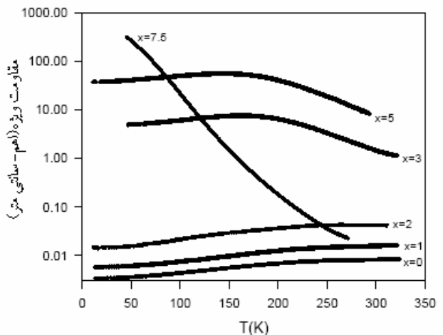
شکل ۱۴. تغییرات مقاومت الکتریکی dc ای نمونه‌های \text{LSMO}/x\text{TiO}_6 در میدان مغناطیسی صفر نسبت به دما.
