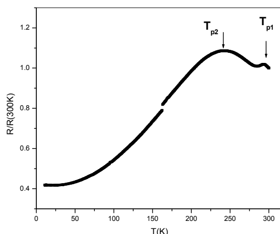
شکل ۲۱. منحنی تغییرات مقاومت الکتریکی dc بر حسب دما در میدان صفر برای نمونه LSMO/xNiO. x=0 .
