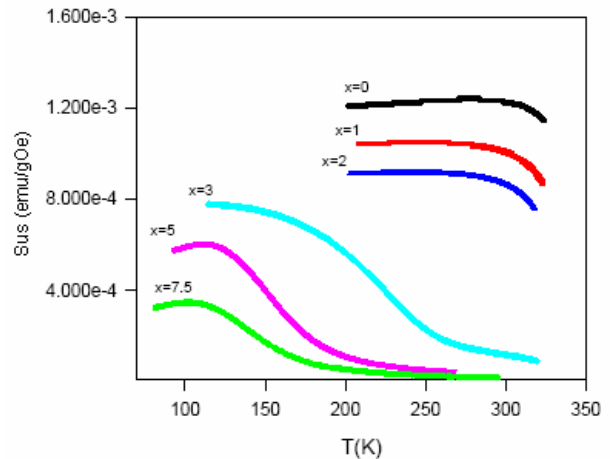
شکل ۱۳. منحنی تغییرات بخش حقیقی پذیرفتاری مغناطیسی ac بر حسب دما برای نمونه‌های \text{LSMO}/x\text{TiO}_6 در میدان ۶ اورستد و بسامد ۳۳۳ هرتز.
