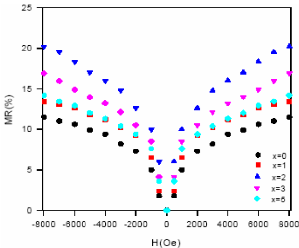
شکل ۱۵. مغناطومقاومت ترکیبات \text{LSMO}/x\text{TiO}_6 در میدان‌های مغناطیسی ۰-۸۰۰۰ اورستد در دمای ۷۷ کلوین.
