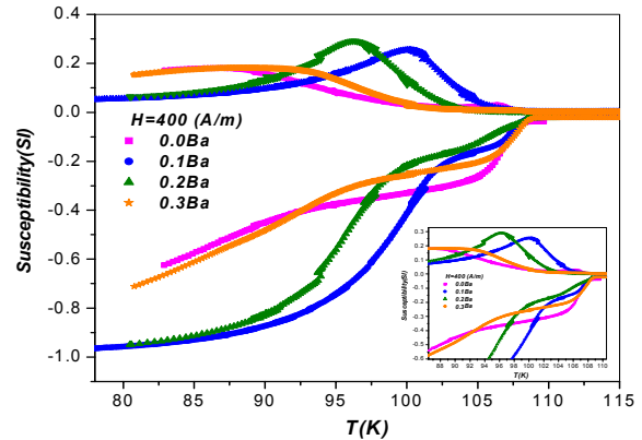
شکل ۳. پذیرفتاری مغناطیسی نمونه‌ها در میدان ۴۰۰ A/m با فرکانس ۳۳۳ Hz.
