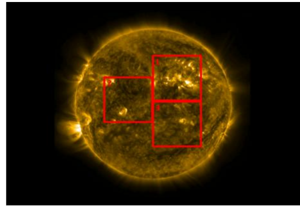
شکل ۱. (رنگی در نسخه الکترونیکی) تصویر قرص کامل خورشید از تلسکوپ اس‌دی‌او در طول موج ۱۷۱ آنگستروم. نواحی ۱، ۲ و ۳ برای تشخیص تاریکی‌های جرم تاجی انتخاب شده است.
