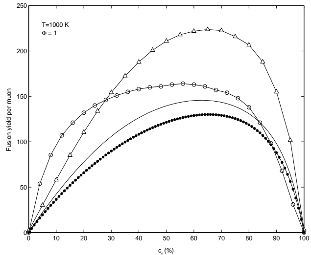
شکل ۴. مقایسه نمودار تغییرات تعداد همجوشی به ازای یک میون نسبت به غلظت تریتوم، از روشهای حل سینماتیک (●) [۴]، حل سینماتیک با در نظر گرفتن اثرات اتمهای فوق حرارتی (Δ) [۸]، منحنی فرمول (۲۹) و شبیه سازی مونت کارلو (○) (کار حاضر) در شرایط T=1000\text{K} و \Phi=1 .
